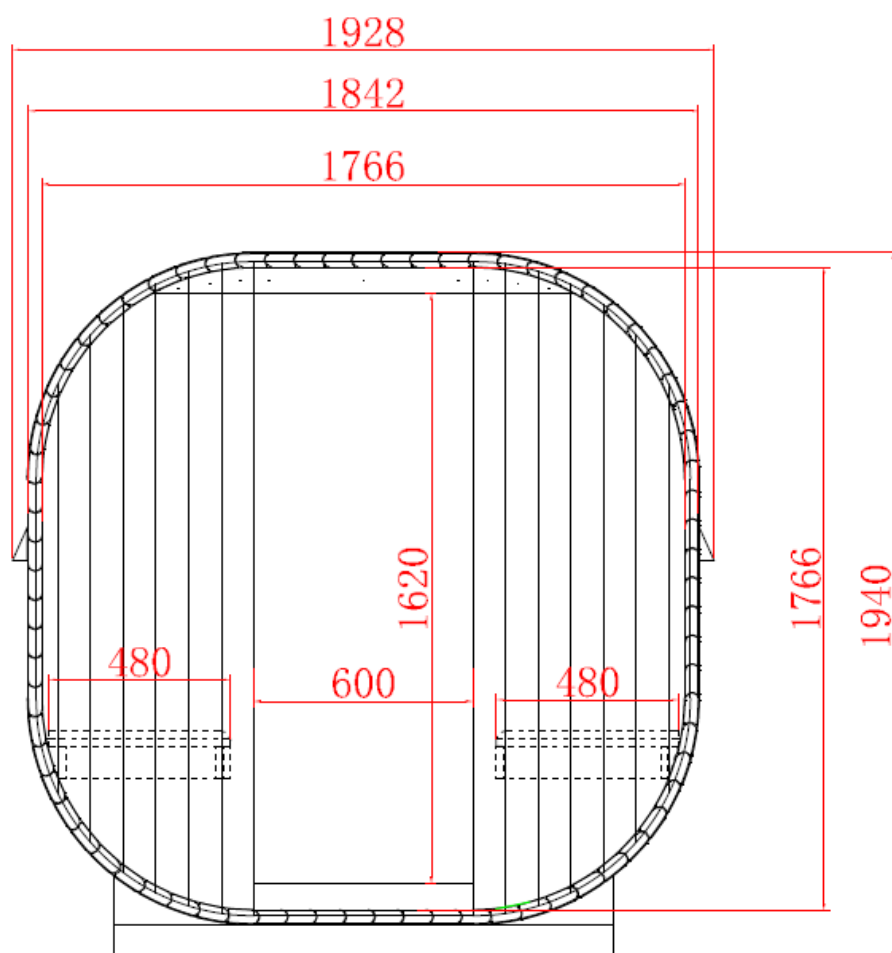
Abbildung 3 Skizze Cube L Deluxe Frontansicht mit Maßen in mm
