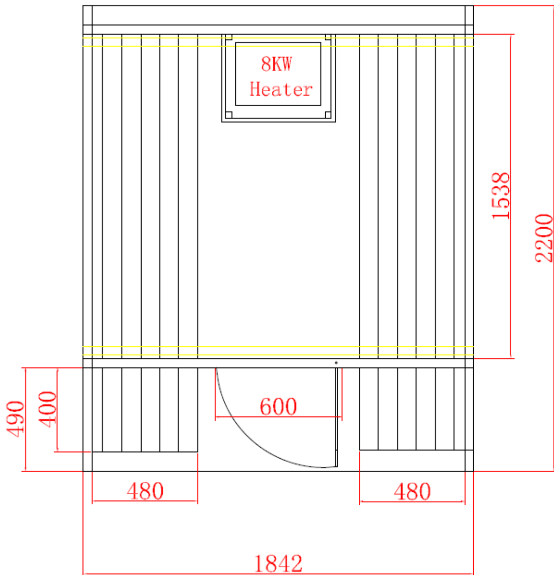
Abbildung 4 Skizze Cube L Deluxe Innenansicht mit maßen in mm
