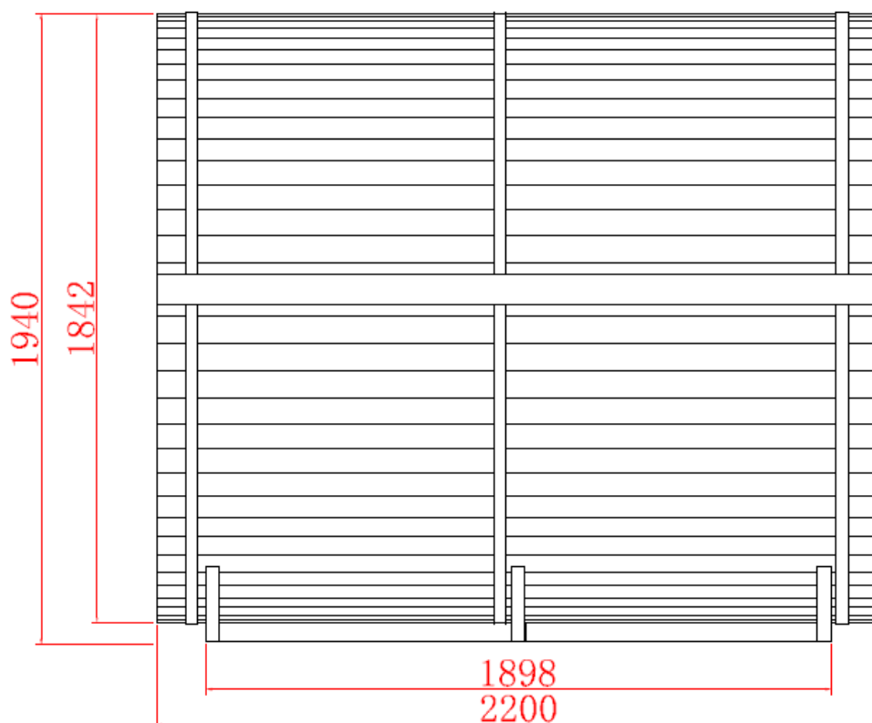
Abbildung 2 Abbildung 2 Skizze Cube L Deluxe Seitenansicht mit Maßen in mm
