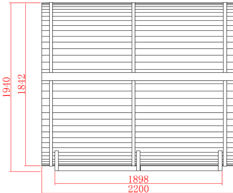
Abbildung 2 Skizze Cube L Deluxe Seitenansicht mit Maßen in mm
